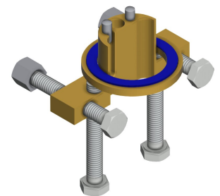
Verdrehsicherung für F55
