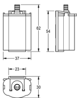
BATTERIEFACH: ZAQCT0003
